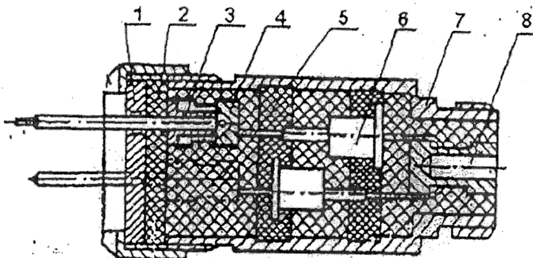
Рис.10 Делитель: 1-Гайка; 2-накладка; 3-сальник; 4-штулка; 5-выходное гнездо; 6-диод; 7-корпус; 8-выводное гнездо.
