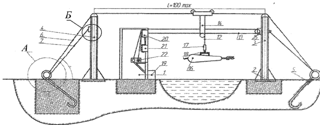
Установка ГР-70
